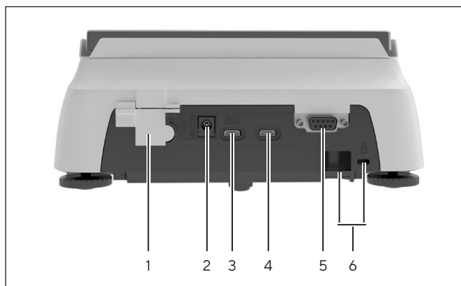
Abb. 2: Präzisionswaage (Rückansicht)
