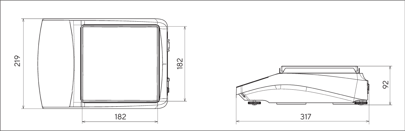
Abb. 8: Gerätemaße in mm
