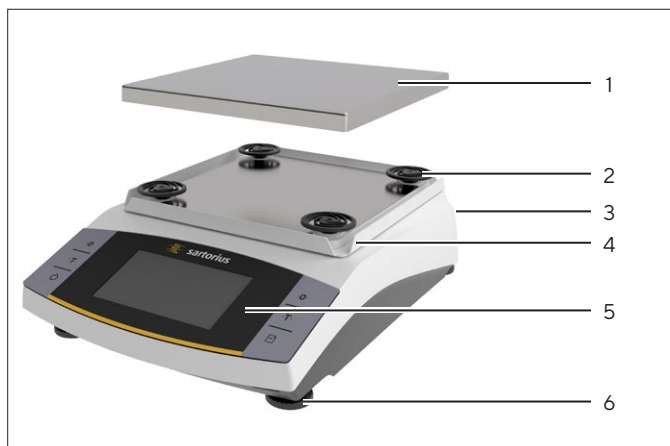
Abb. 1: Präzisionswaage (Vorderansicht)
